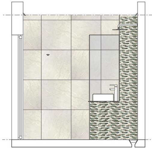
ELEVATION G
